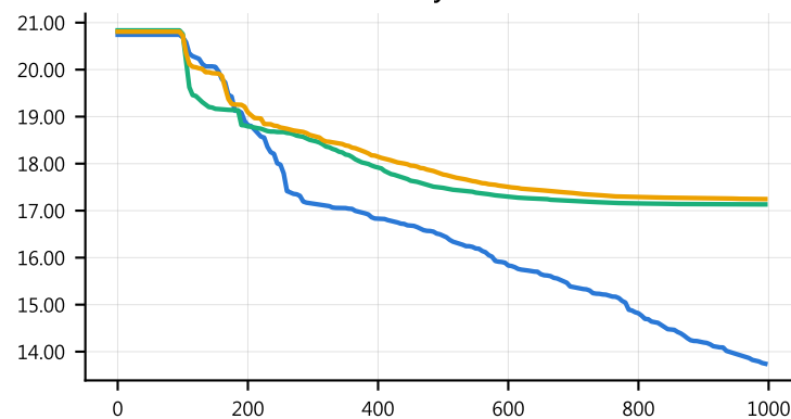
Ellipsoid · 50D
