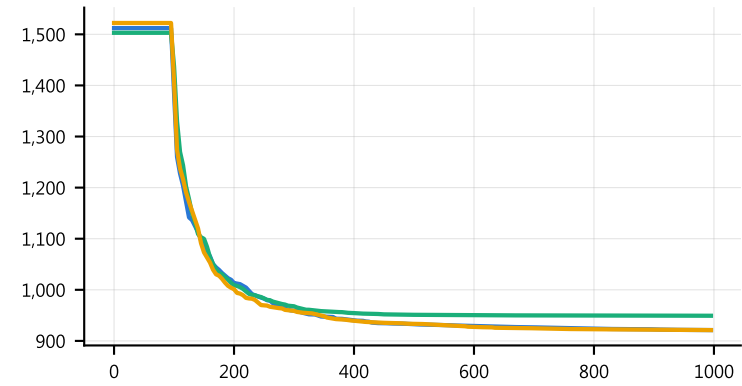
Rosenbrock · 50D
