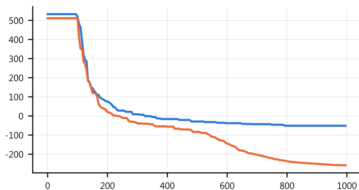
SRR · 30D
