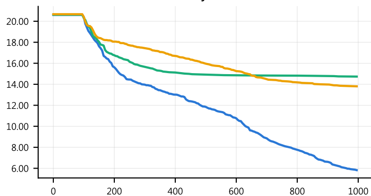
Ellipsoid · 30D
