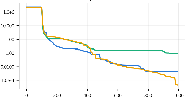
Griewank · 30D
