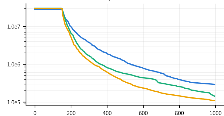
Griewank · 100D
