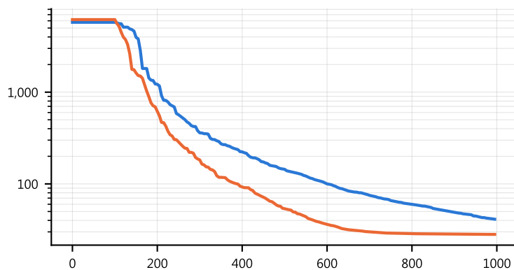
SRR · 30D
