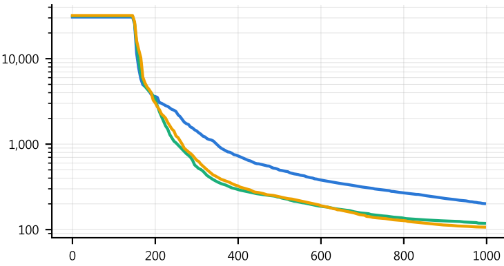
Rosenbrock · 100D
