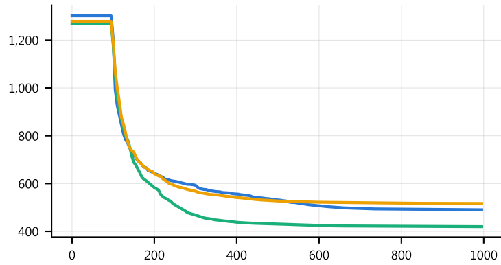
RHC2 · 50D
