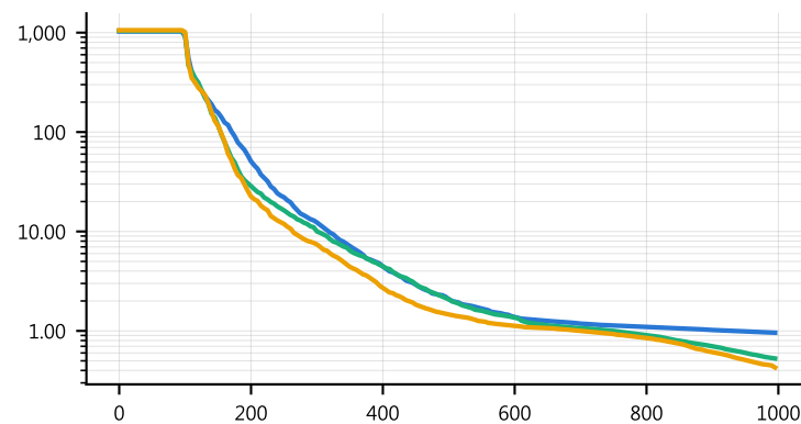
Griewank · 50D
