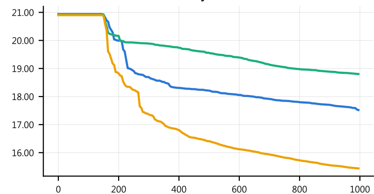
Ellipsoid · 100D
