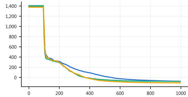
SRR · 50D
