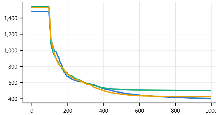
Rosenbrock · 30D
