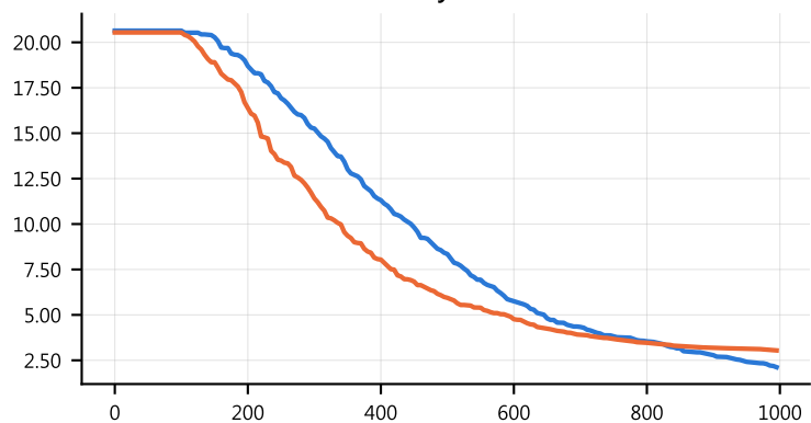
RHC1 · 30D
