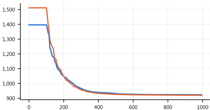
RHC2 · 30D
