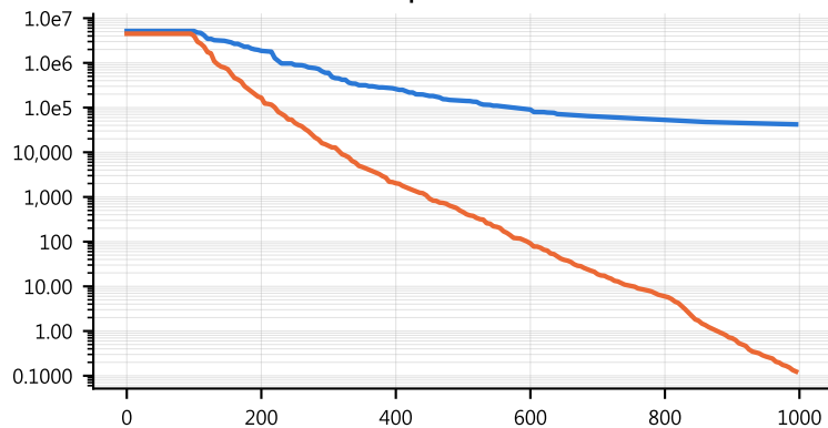
Griewank · 30D
