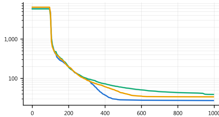
SRR · 30D
