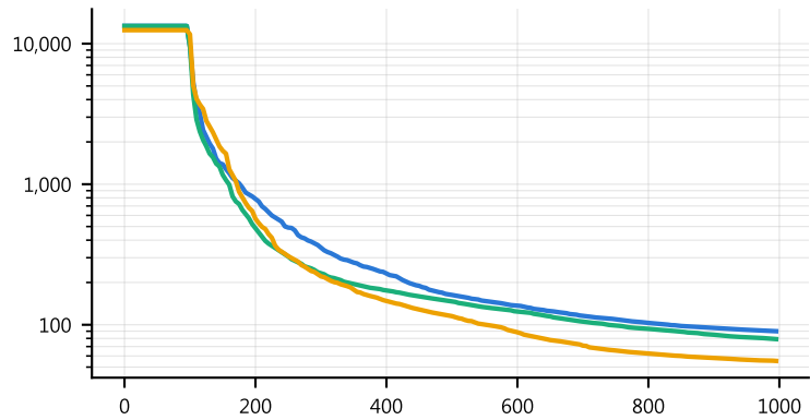
SRR · 50D
