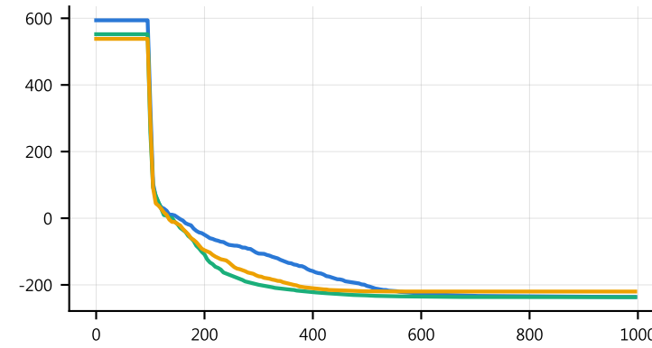
SRR · 30D
