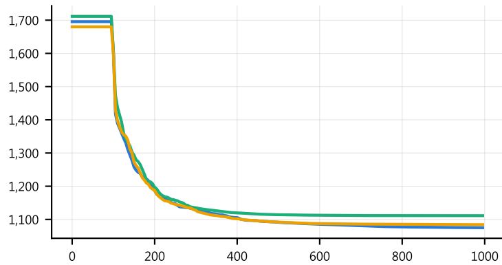
Rosenbrock · 100D
